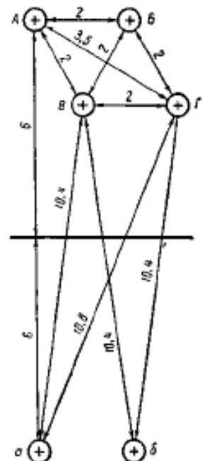
Рис. 14. Схема расположения проводов
